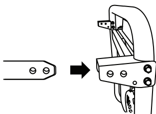
FIGURA 11: Inserte la barra de la manija en el soporte
