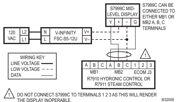
Fig. 11. S7999C wiring diagram.
