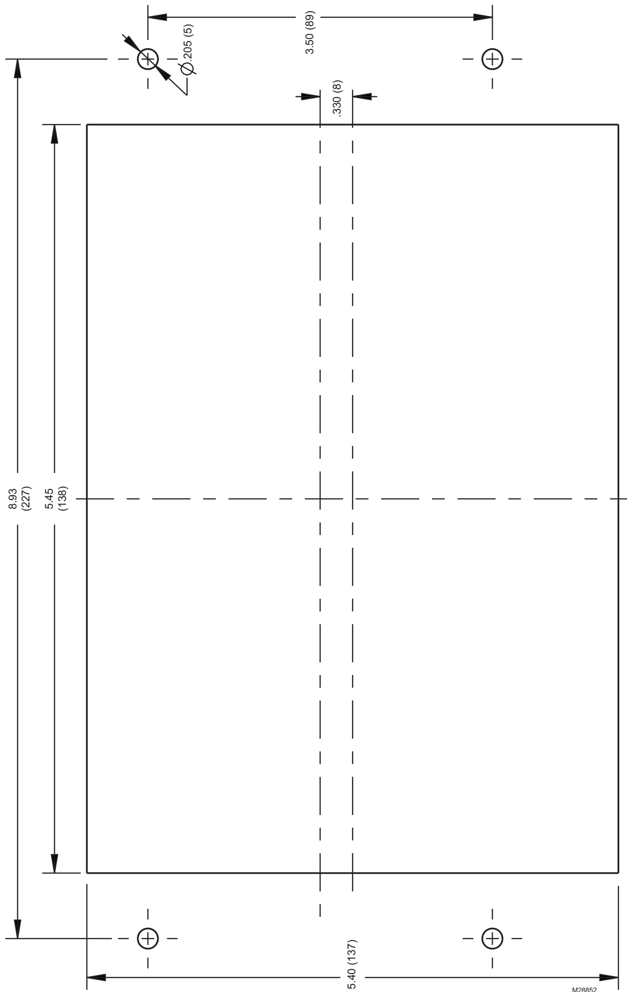
Fig. 121. S7999C front-mount template.
