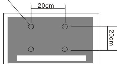
Dimension de quatre trous de montage: Vis M4
