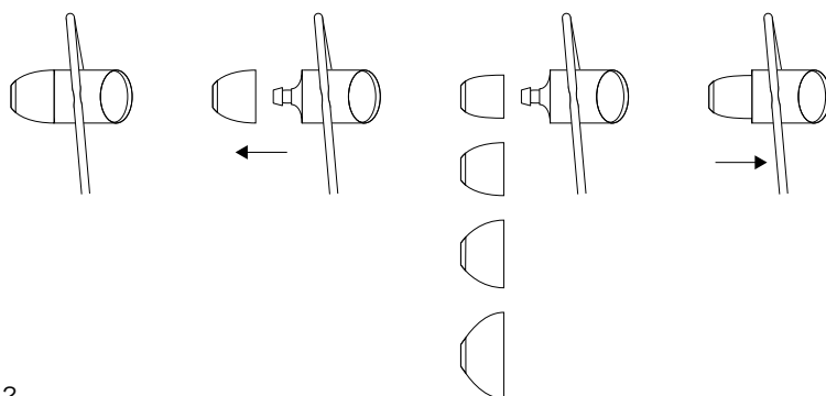
図2 イヤーピースの交換方法
