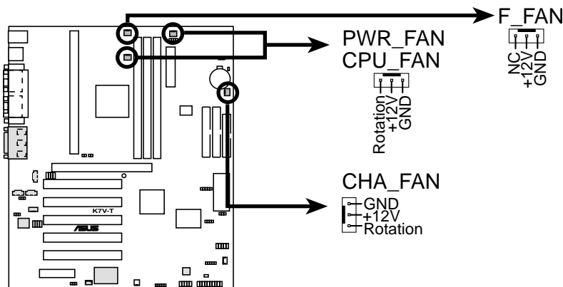
K7V-T 12-Volt Cooling Fan Power
