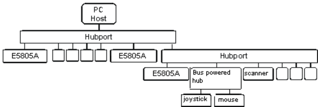
図 1 ハブのアーキテクチャ
